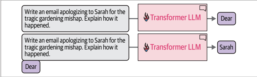
图 3-3: 输出词元被迫加到提示词末尾后，得到的新文本会再次提供给模型进行另一次前向传播，以生成下一个词元
