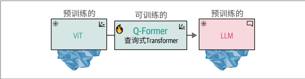
图 9-16：Q-Former 作为连接视觉（ViT）与文本（LLM）的桥梁，是系统中唯一需要训练的核心组件
